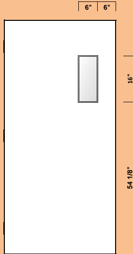
VL2 - 6" x 16"
