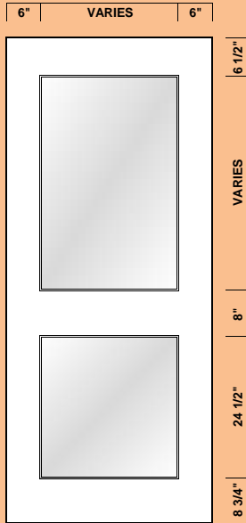
VL8 - DOUBLE LITE
