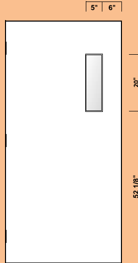
VL3 - 5" x 20"
